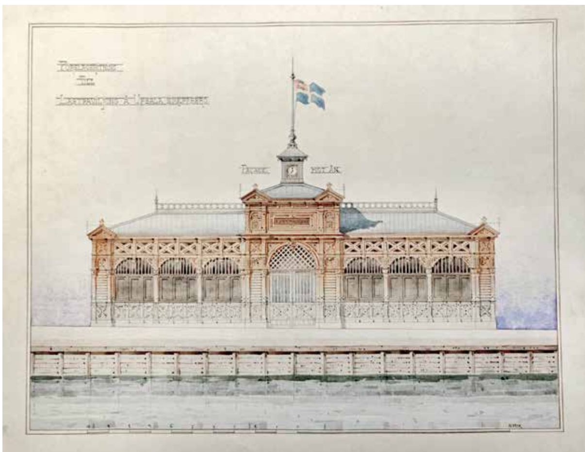
Odaterad och osignerad ritning över "Lastpaviljong å Upsala Skeppsbro", troligen utförd 1875 av stadsingenjör Ludwig Wåhlberg. Uppsala stadsarkiv.
